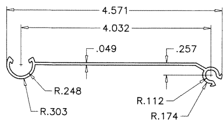
SLAT 6063-T6
