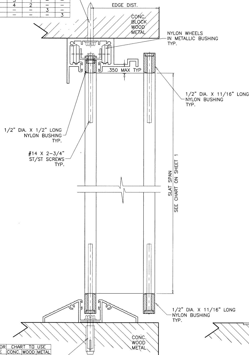
SECTION A-A
